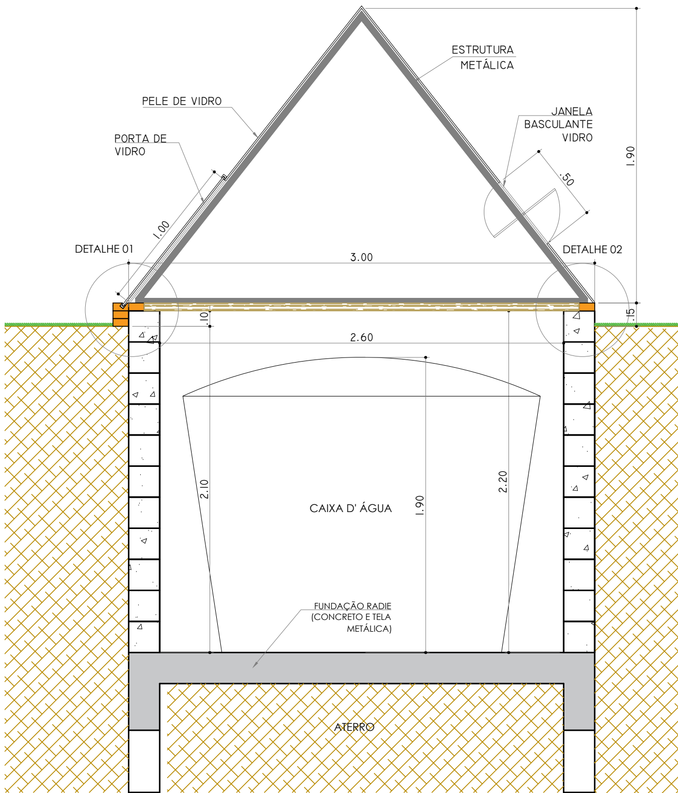
CORTE ESCALA 1:25
